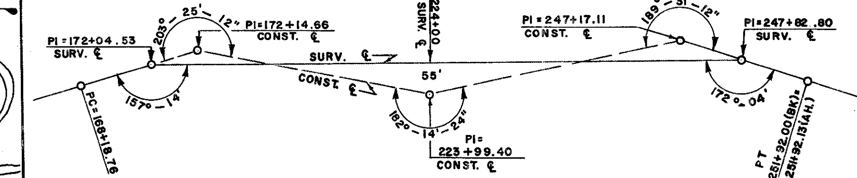
LINE SHIFT DIAGRAM STA. 168+18.76 TO STA. 251+92.13
