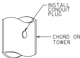
CONDUIT PLUG DETAIL
